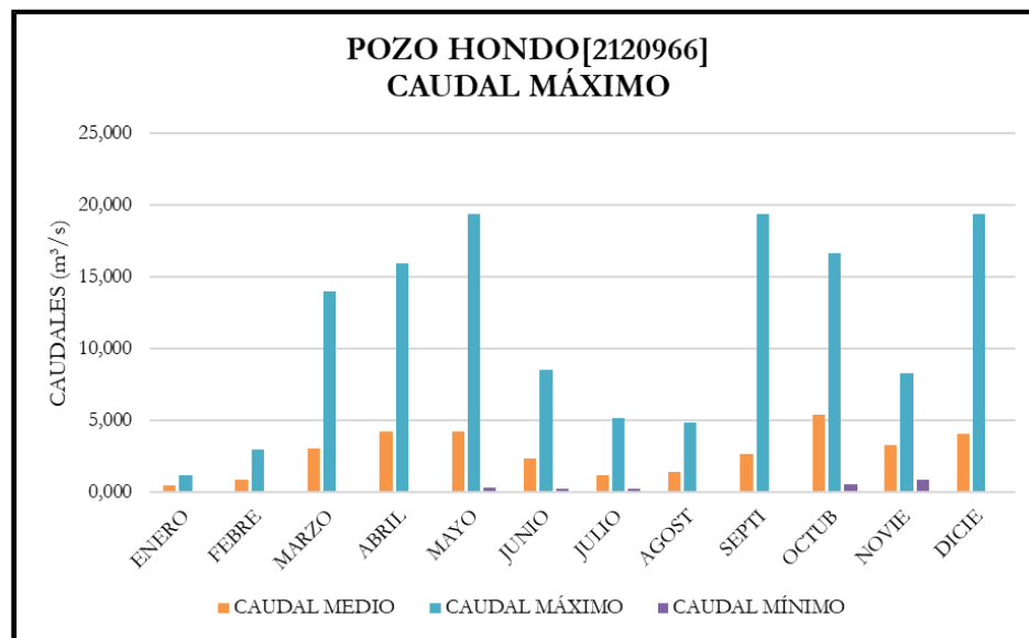
Ilustración 169. Caudales máximos estación Pozo Hondo [2120966].
