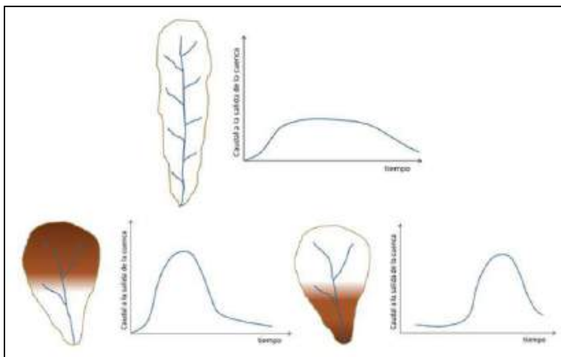
Ilustración 145. Influencia de la configuración de la red hidrológica en las descargas.
