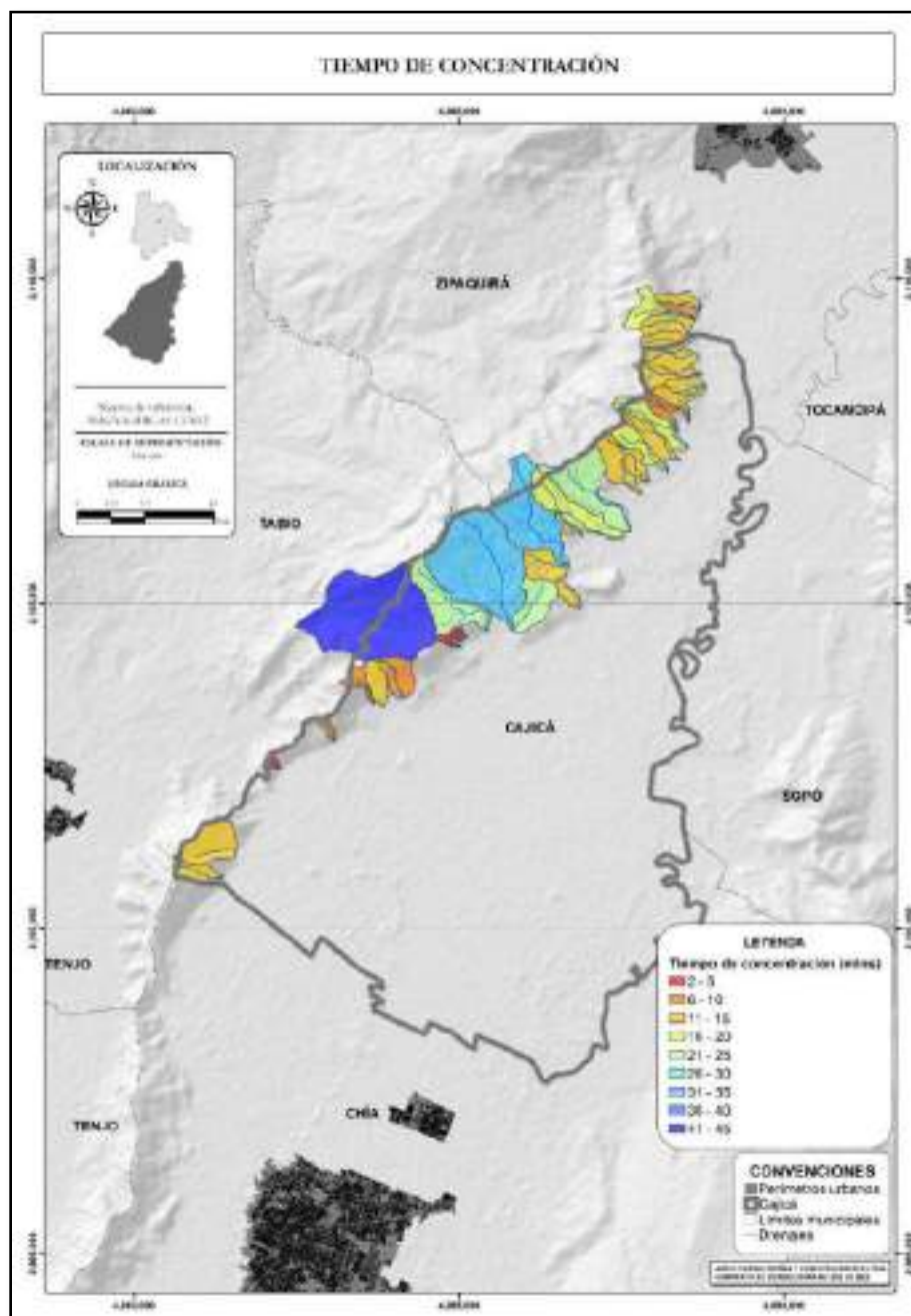
Ilustración 158. Tiempo de concentración de las microcuencas.
