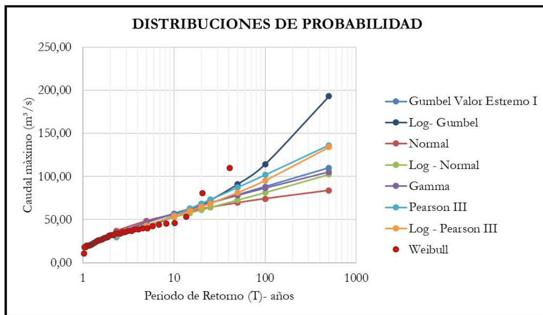
Ilustración 185. Ajuste distribuciones de probabilidad estación Puente Vargas [2120734].
