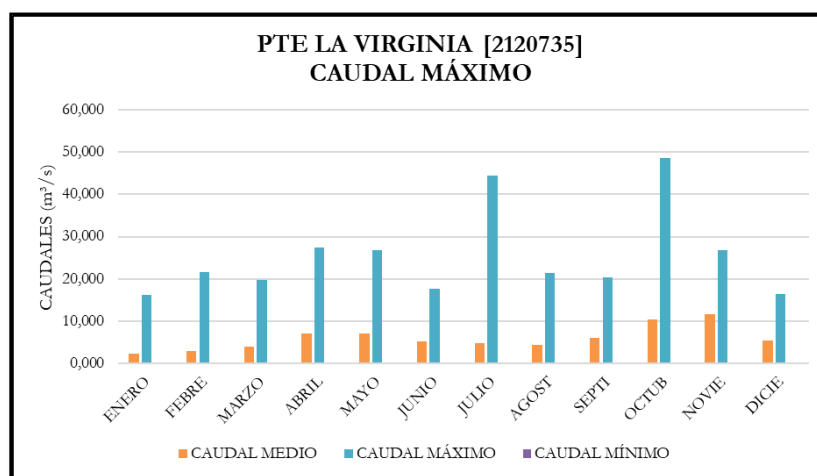
Ilustración 171. Caudales máximos estación Puente La Virginia [2120735].
