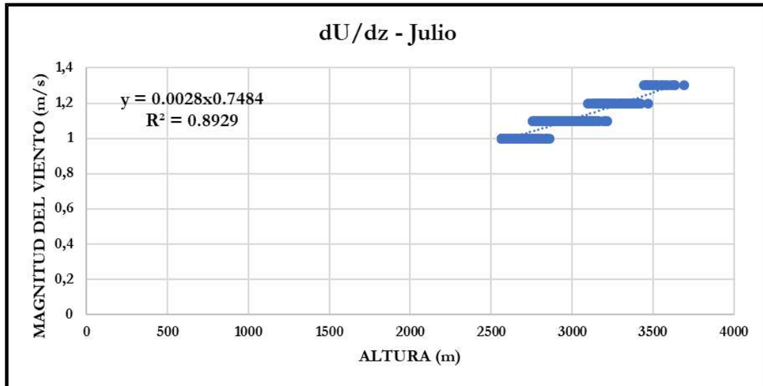
Ilustración 19. Función de correlación de la magnitud del viento con la altura para el mes de julio
