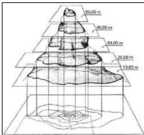
Ilustración 116. Modelo de elevación derivado en curvas de nivel.
