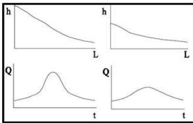
Ilustración 154. Hidrogramas en relación perfil altimétrico cauce principal.
