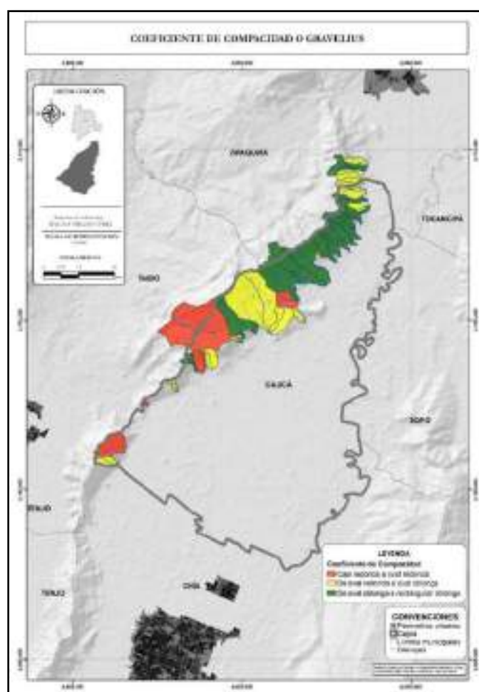
Ilustración 142. Coeficiente de Compacidad o Gravelius.
