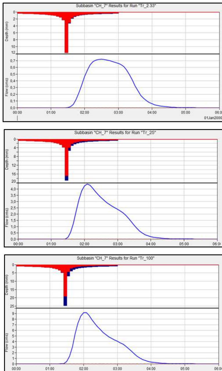
Ilustración 190. Mosaico de hidrogramas unitarios para los periodos de retorno de 2.33, 25 y 100 años.
