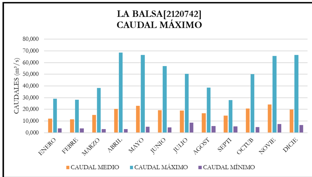
Ilustración 167. Caudales máximos estación La Balsa Chía [2120742].
