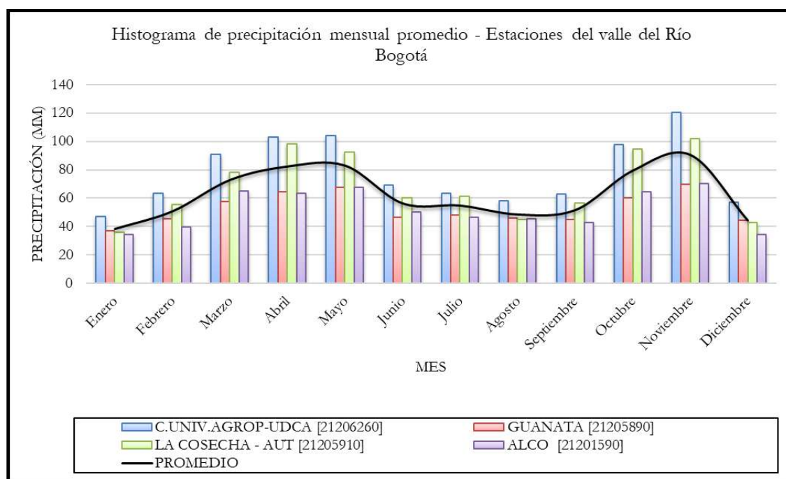
Ilustración 10. Histograma de precipitaciones mensuales multianuales en las estaciones ubicadas sobre el valle del Río Bogotá.
