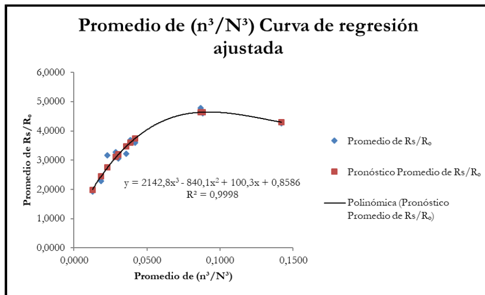
Ilustración 24. Regresión ajustada para el cálculo de la radiación solar
