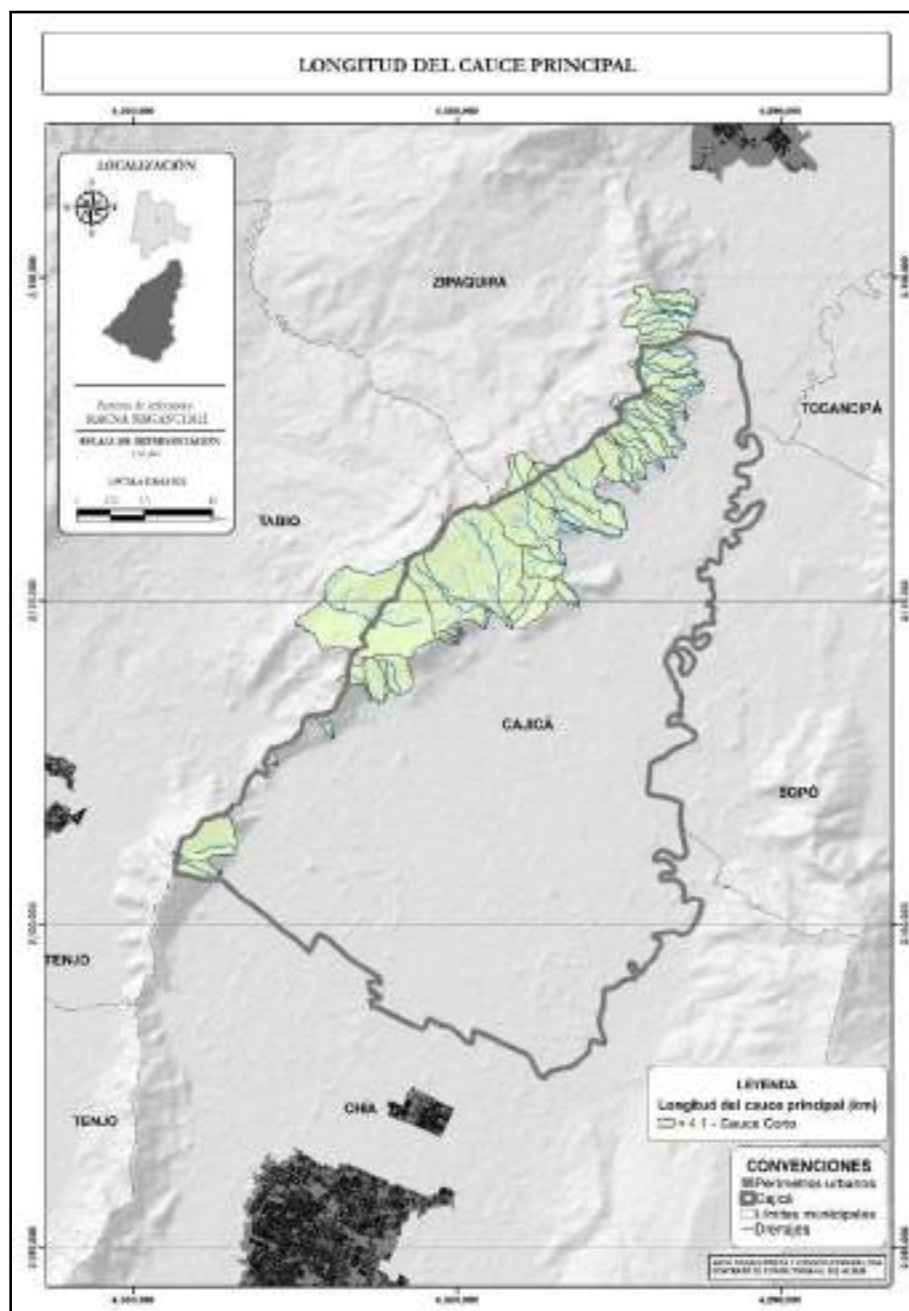
Ilustración 139. Longitud del cauce principal (kilómetros).
