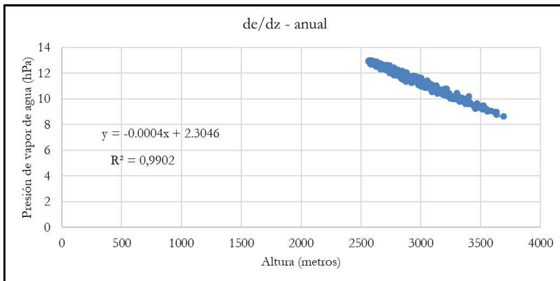
Ilustración 26. Relación de la Presión de Vapor de Agua con la altura.
