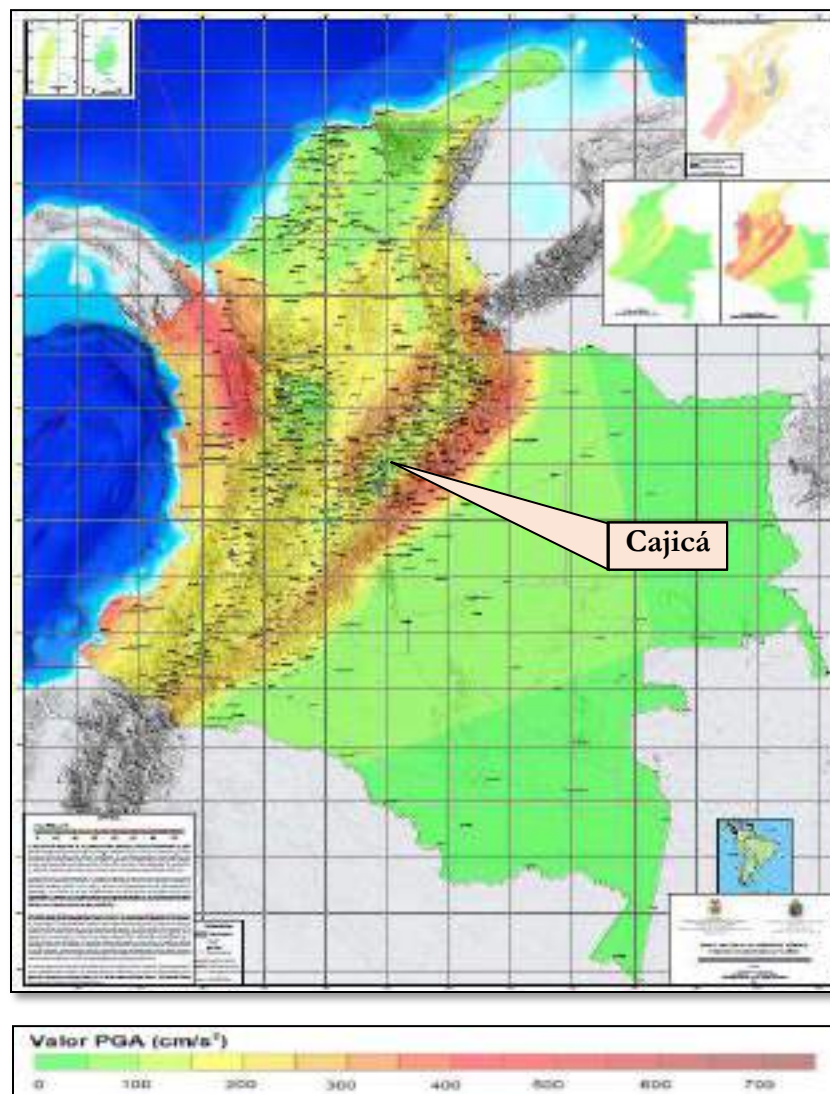
Ilustración 132. Zonificación sísmica para un período de retorno de 475 años.
