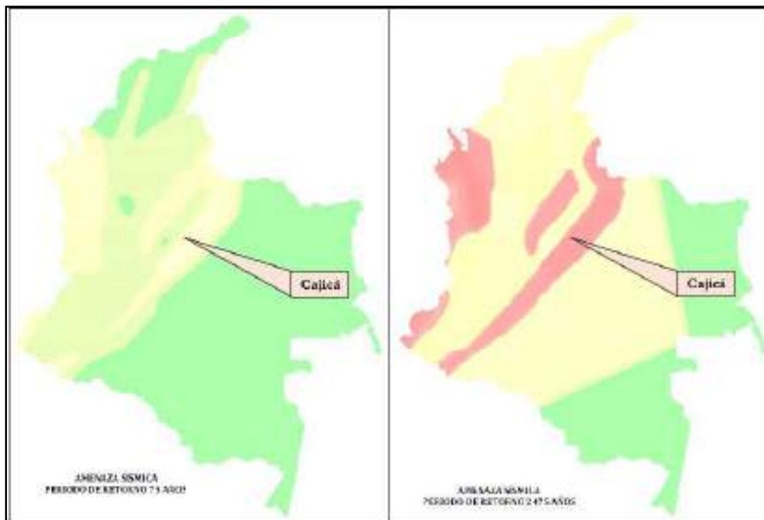
Ilustración 131. Mapa de sismicidad para períodos de retorno de 75 años (izq.) y 2475 años.
