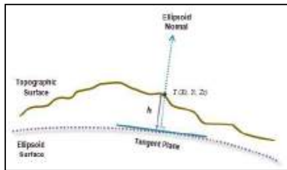
Ilustración 124. Ejemplo cálculo y comportamiento geodésico I.
