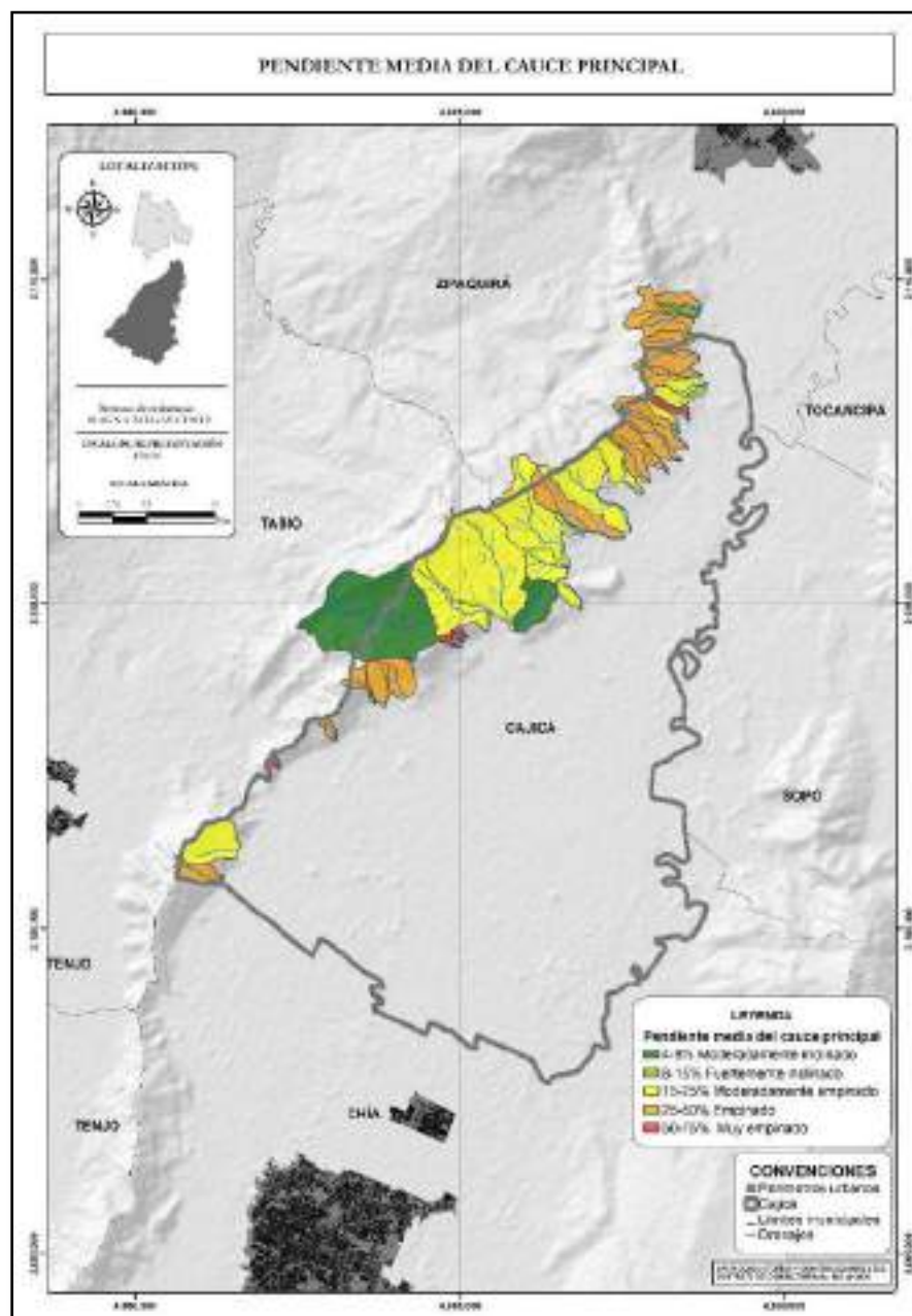
Ilustración 153. Pendiente media del cauce principal.
