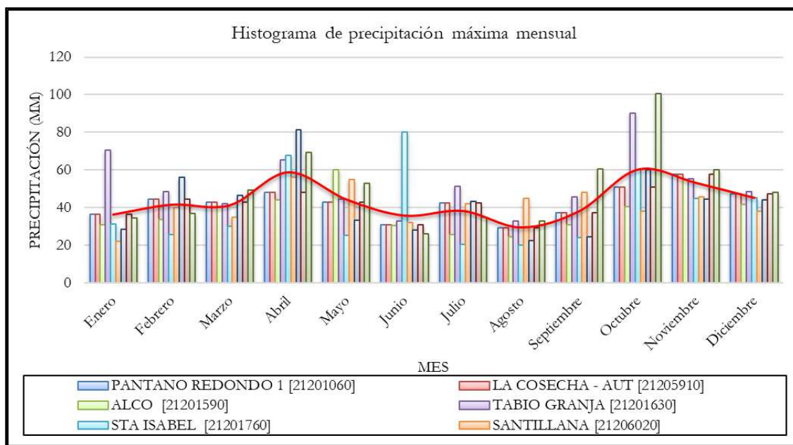
Ilustración 11. Histograma de precipitaciones máximas mensuales históricas en las estaciones evaluadas.
