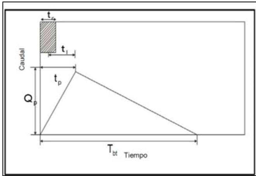
Ilustración 188. Hidrograma Unitario Triangular del SCS.
