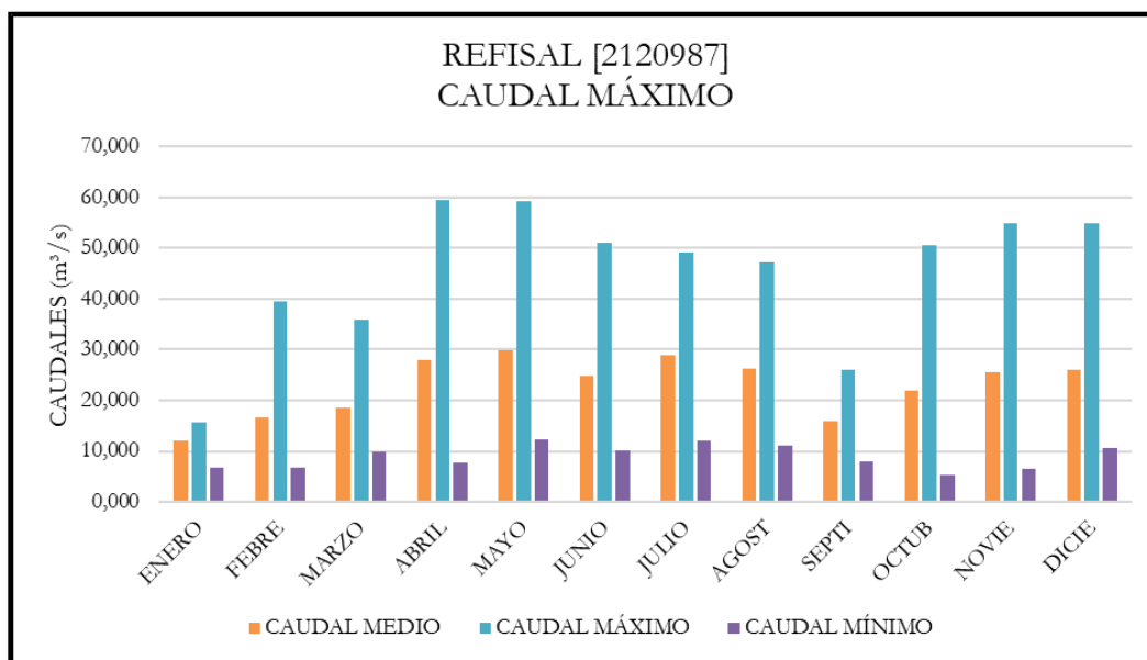
Ilustración 165. Caudales máximos estación Refisal [2120987].
