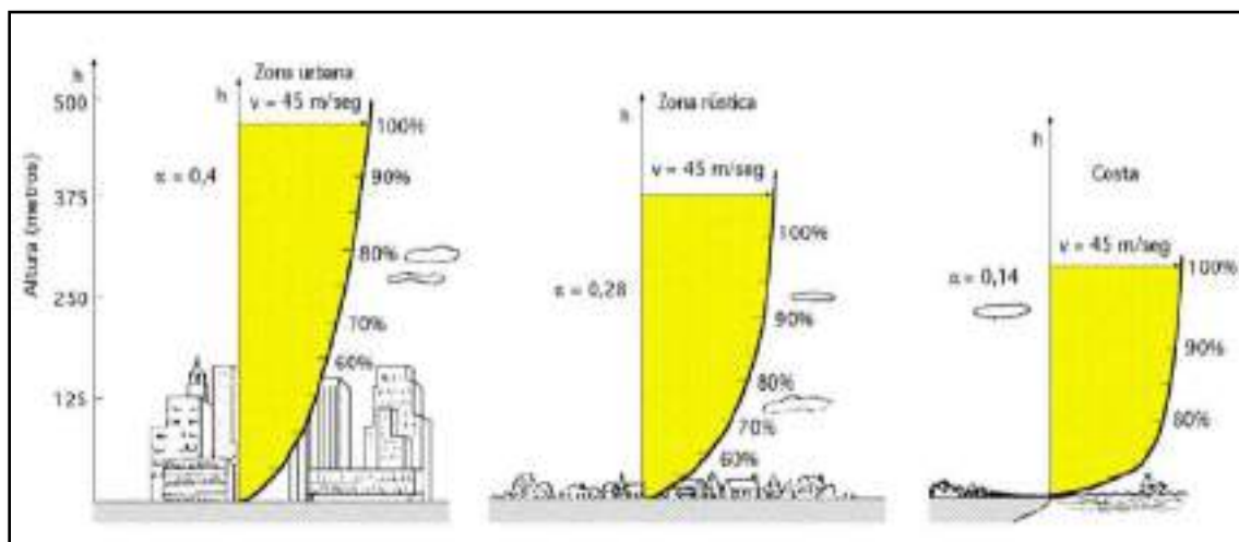
Ilustración 18. Perfiles de velocidad del viento en diferentes escenarios.
