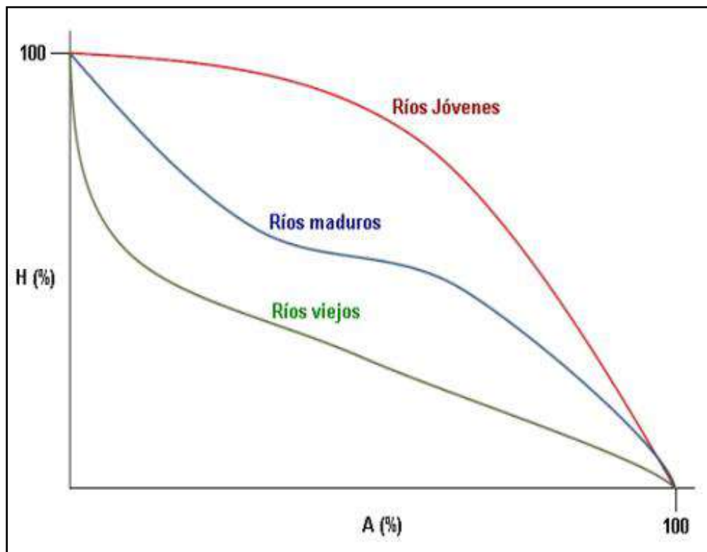
Ilustración 148. Clasificación de ríos a partir de la curva hipsométrica.
