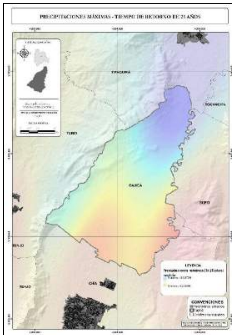
Ilustración 162. Precipitaciones máximas esperadas para periodos de retorno de 25 años.
