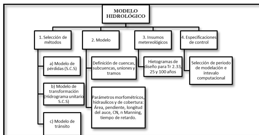
Esquema 7. Modelo hidrológico HEC-HMS.
