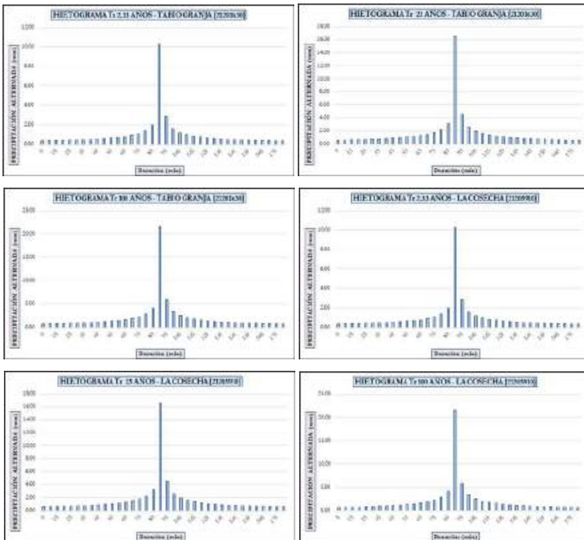
Ilustración 186. Mosaico de Hietogramas de diseño de las estaciones “TABIO GRANJA [21201630]” y “LA COSECHA – AUT [21205910]” para periodos de retorno de 2.33, 25 y 100 años.
