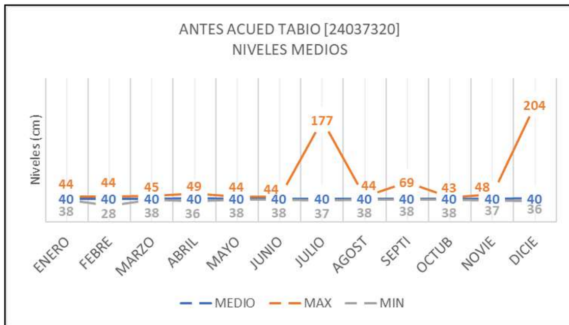
Ilustración 184. Niveles máximos estación Antes Acueducto Tabio [2120923].
