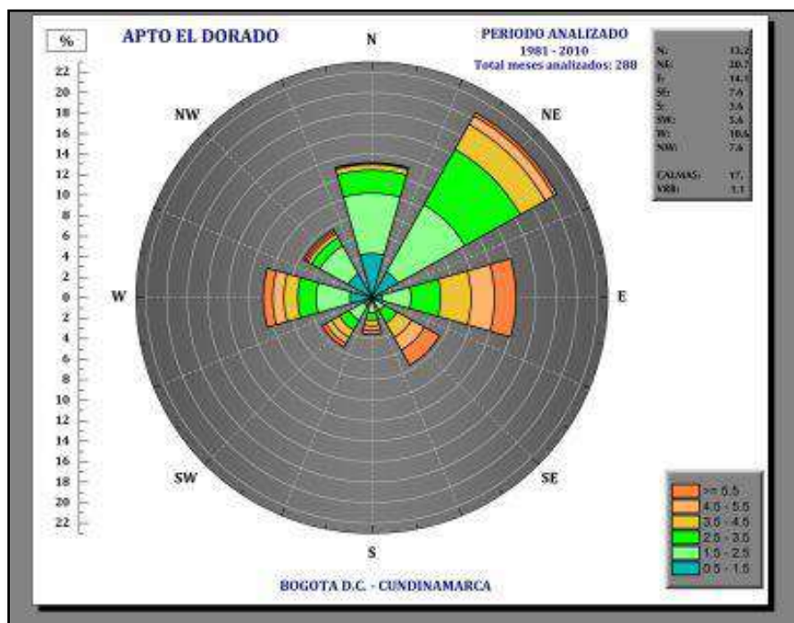
Ilustración 21. Roseta de vientos de la estación "APTO EL DORADO"
