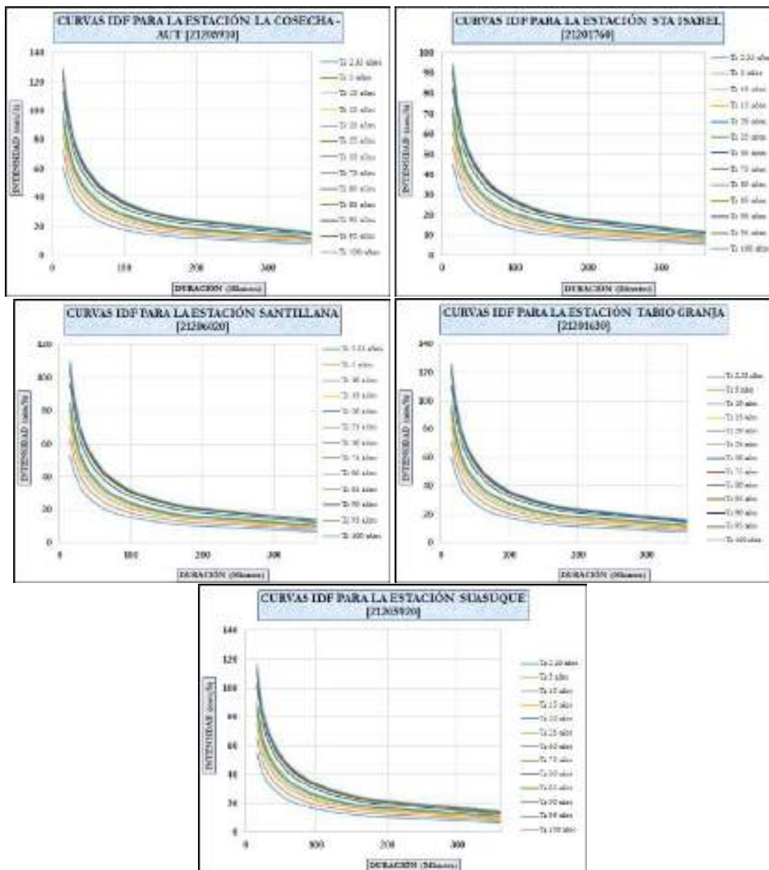
Ilustración 159. Mosaico de Curvas de Intensidad, Duración y Frecuencia (IDF) para las estaciones de análisis.
