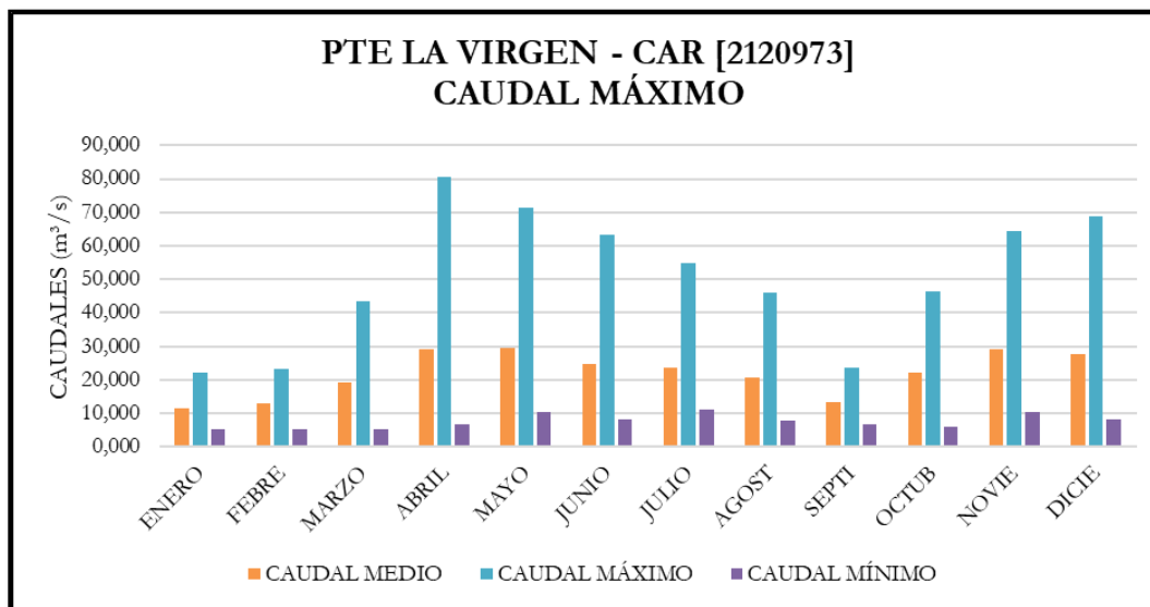
Ilustración 168. Caudales máximos estación Puente La Virgen [2120973].
