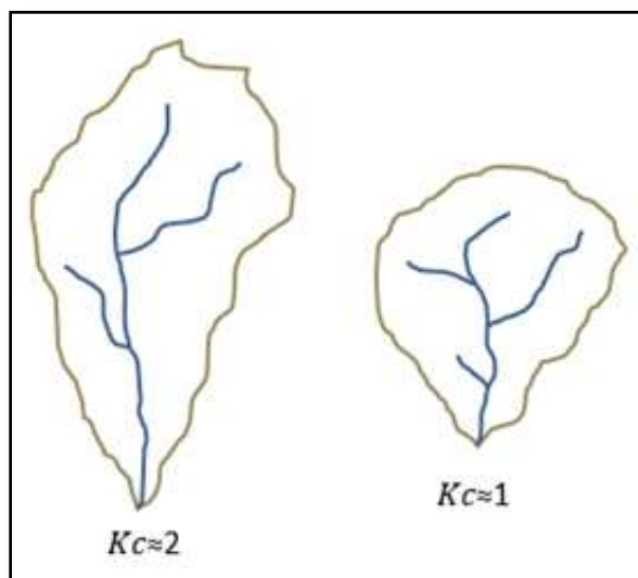
Ilustración 143. Comparación de la forma de las cuencas con el Coeficiente de Compacidad.
