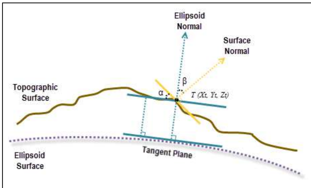
Ilustración 126. Ejemplo cálculo y comportamiento geodésico II.
