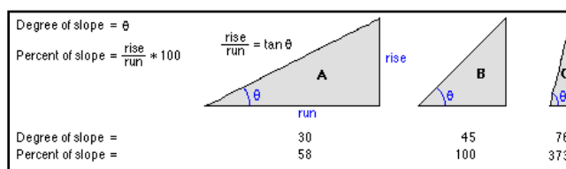
Ilustración 120. Modelo explicativo de pendientes de suelo.
