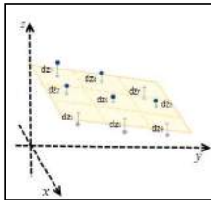
Ilustración 125. Ejemplo ajuste de mínimos cuadrados.
