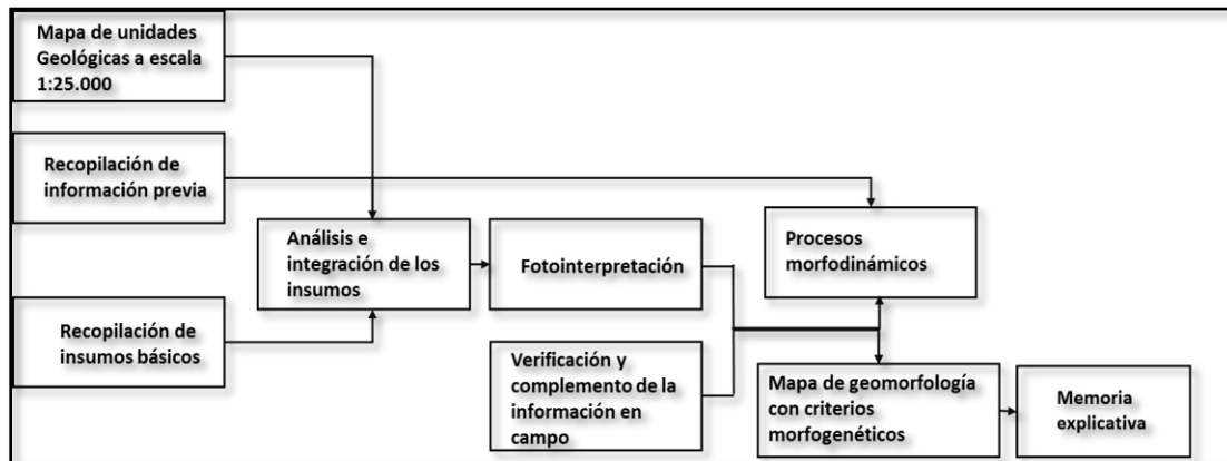
Esquema 6. Proceso metodológico para la obtención del mapa geomorfológico a escala 1:25.000.
