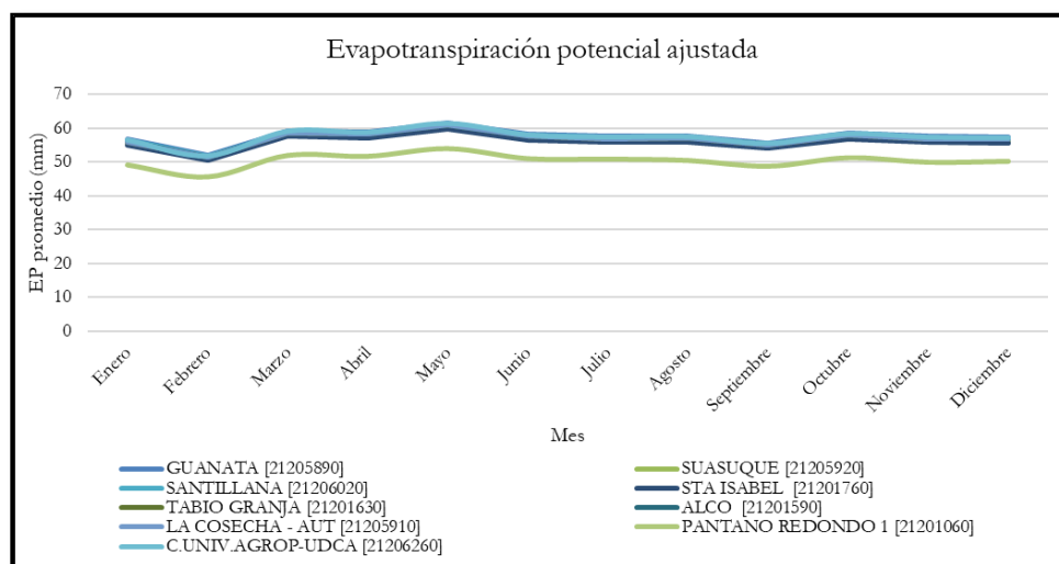
Ilustración 31. Evapotranspiración mensual promedio de las estaciones de análisis.
