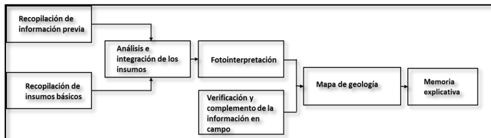
Esquema 4. Proceso Metodológico para la obtención del mapa geológico a escala 1:25.000.
