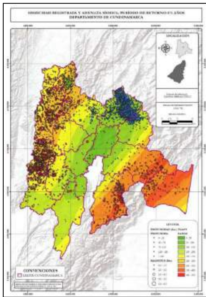
Ilustración 133. Sismicidad registrada y amenaza sísmica con período de retorno 475 años en el departamento de Cundinamarca.
