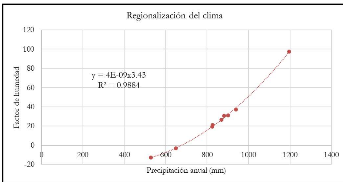
Ilustración 33. Gráfica de la relación del factor de humedad y la precipitación anual.
