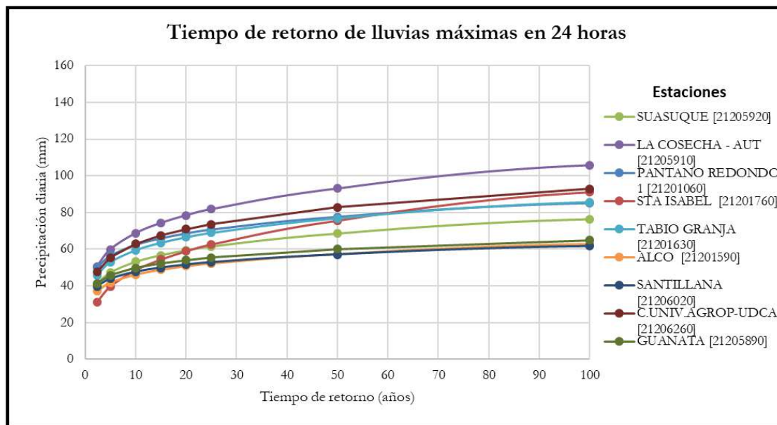
Ilustración 160. Lluvias máximas para periodos de retorno de 2.33 a 100 años.
