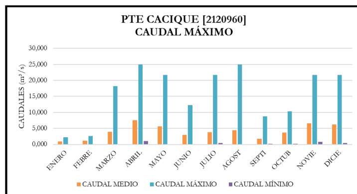
Ilustración 172. Caudales máximos estación Puente Cacique [2120960].
