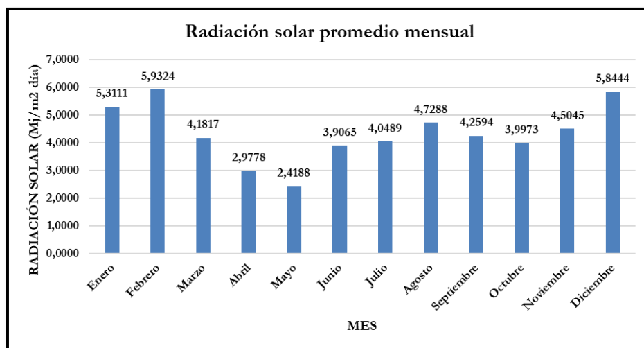
Ilustración 23. Radiación solar diaria promedio mensual histórica
